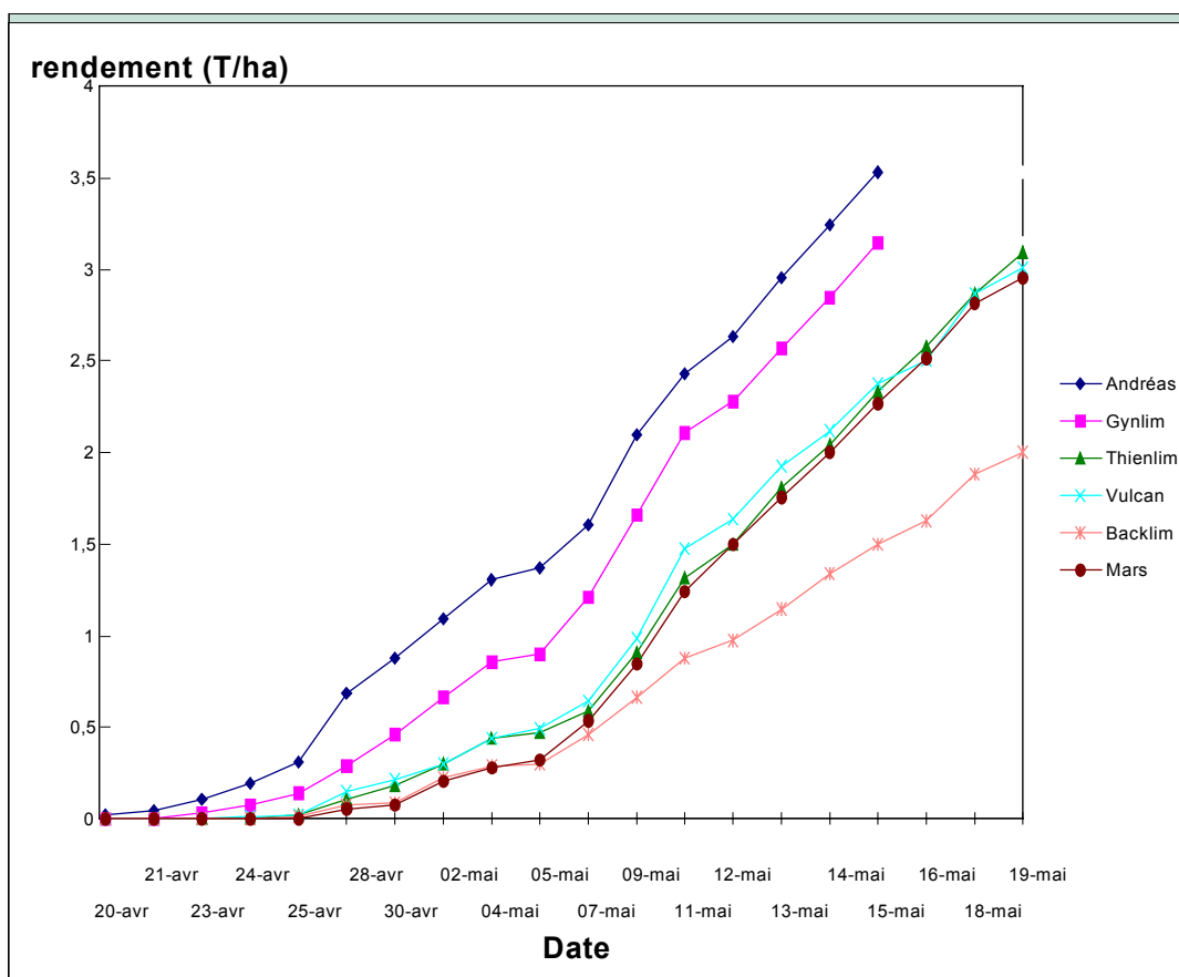
Figure 16 : rendement cumulé par variété
