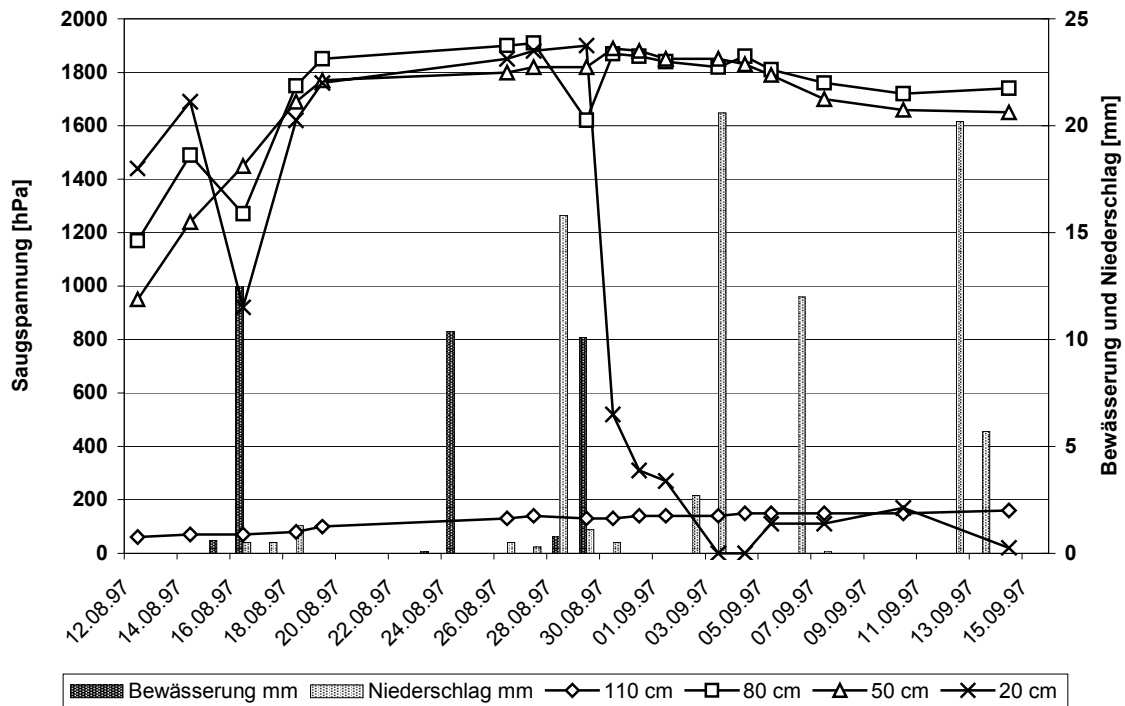
Figure 7 : valeurs de tensions du sol pour l'irrigation aérienne
