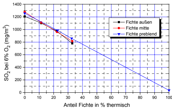
Abb.7: \text{SO}_2 -Emissionen in Abhängigkeit des Biomasseanteils
