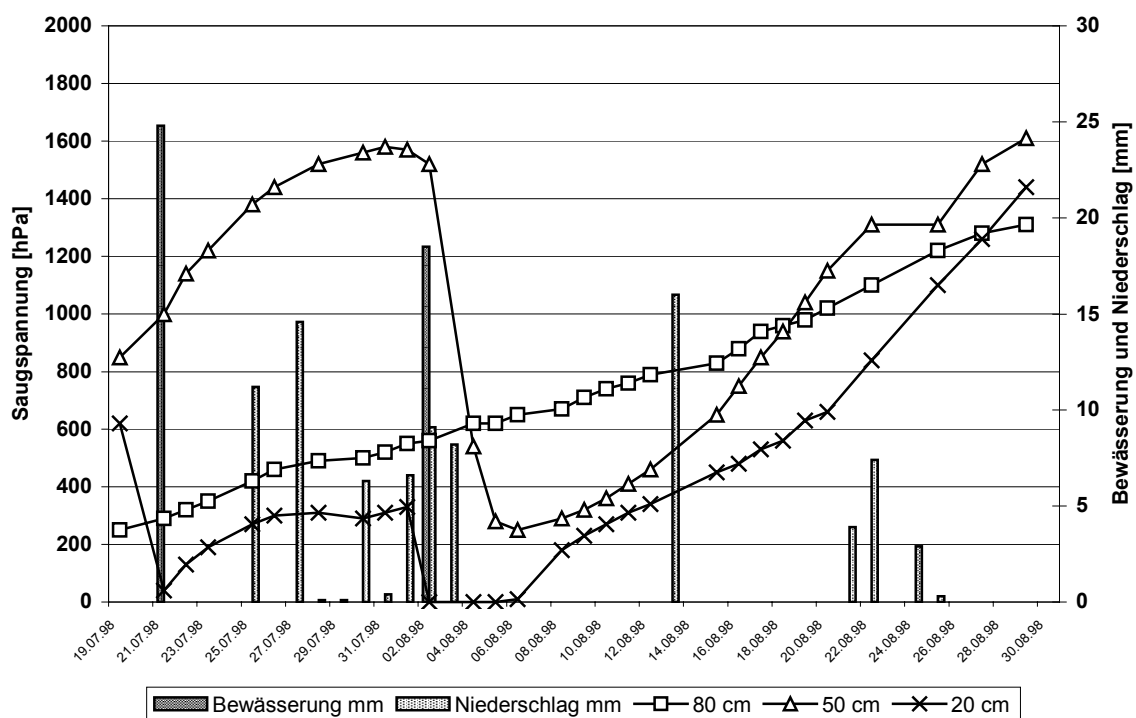
Bild 12: Saugspannungswerte bei Überkopfbewässerung
