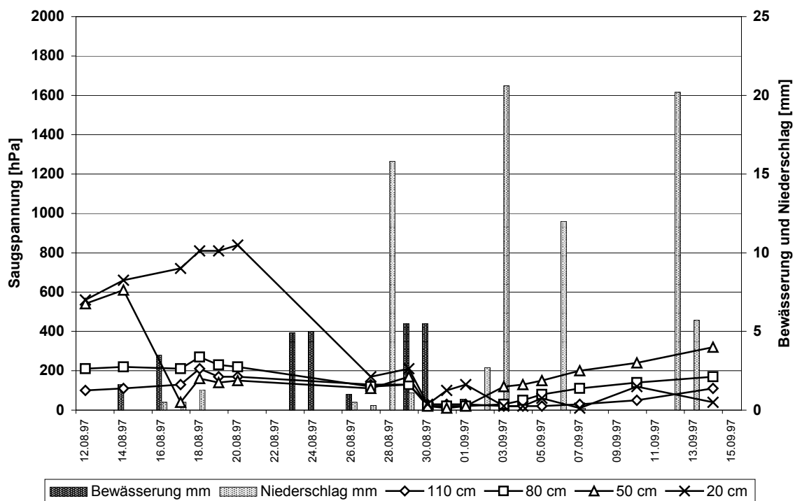
Bild 6: Saugspannungswerte im Boden bei Unterflurbewässerung (Parzelle 16, RAM)
